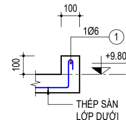
CHI TIẾT KK
