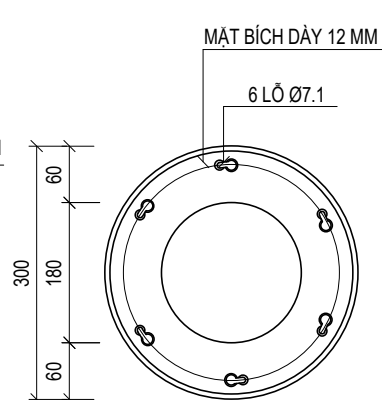
CHI TIẾT ĐỈNH CỌC TỈ LỆ: 1/10
