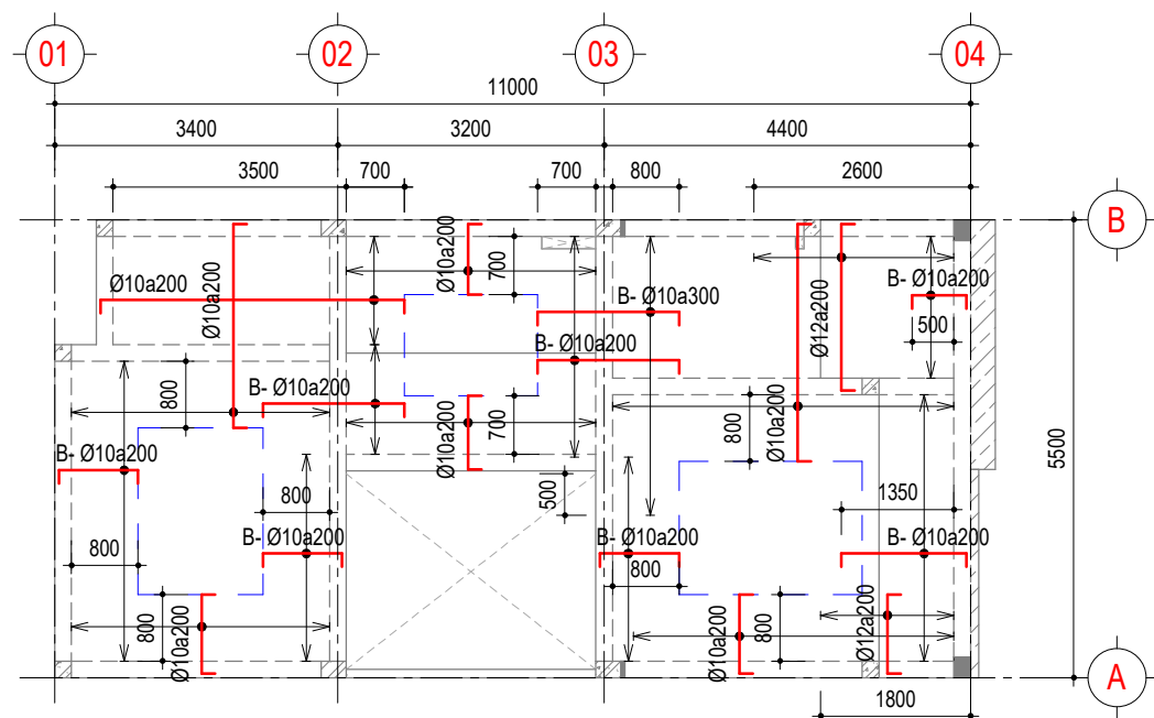
MẶT BẰNG THÉP SÀN TẦNG 3-LỚP TRÊN
