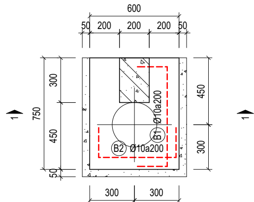
MÓNG M1 (SL=2)
