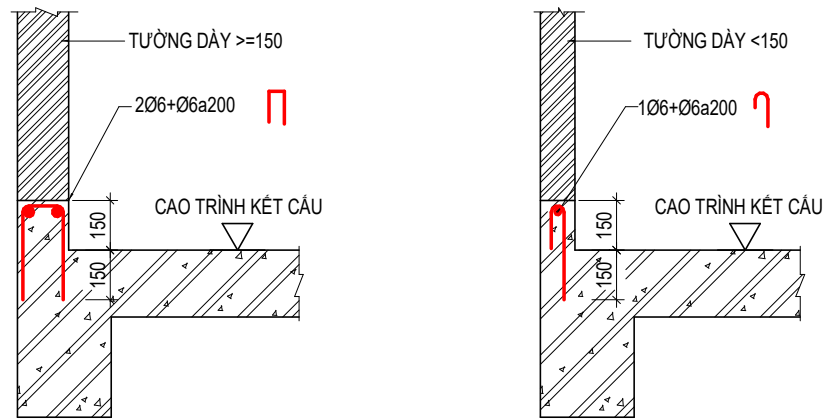
DOC THEO ĐẦU DẦM TƯỜNG DÀY >=150
