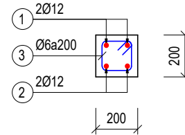
DẪN LT1 (SL=1; L=9300) TL: 1/25
