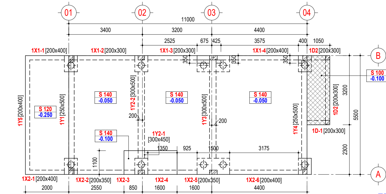
MẶT BẰNG DẦM SÀN - TẦNG 1
