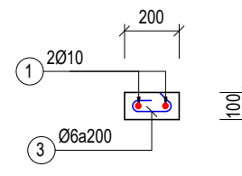
DẪN LT2 (SL=1; L=9600) TL: 1/25
