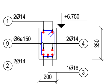
MC 8-8 3X1 (TL: 1/25)
