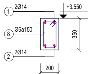
MC 1-1 2X1 (TL: 1/25)
