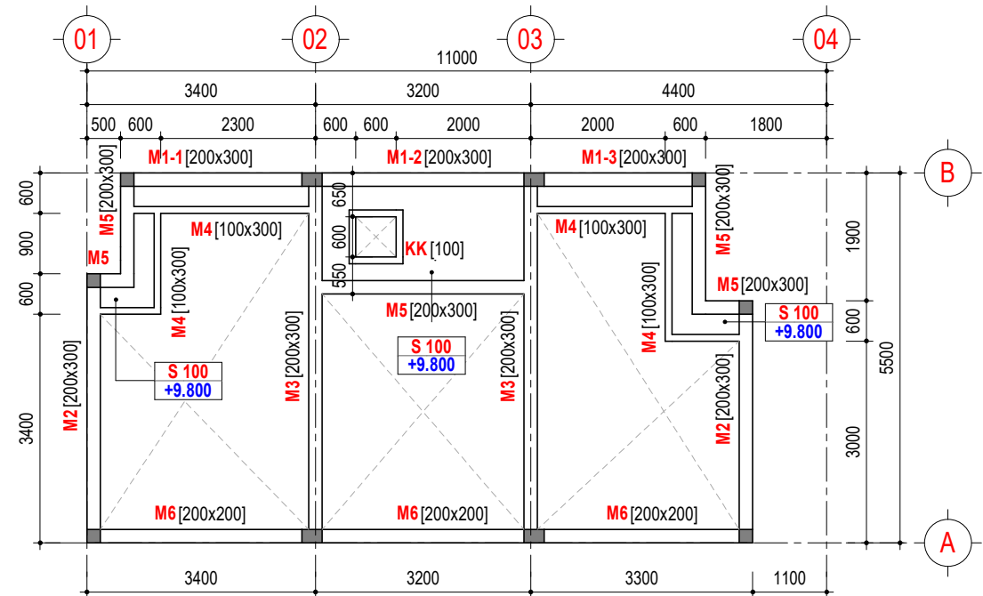
MẶT BẰNG DẦM SÀN - MÁI
