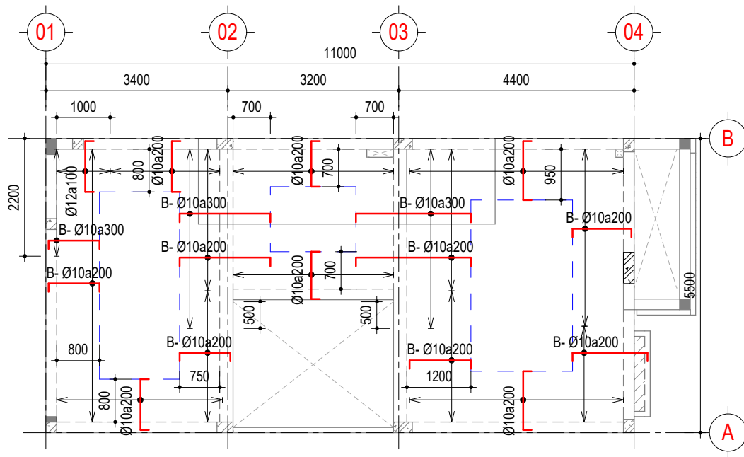
MẶT BẰNG THÉP SÀN TẦNG 2-LỚP TRÊN
