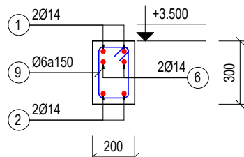
MC 5-5 2X1 (TL: 1/25)
