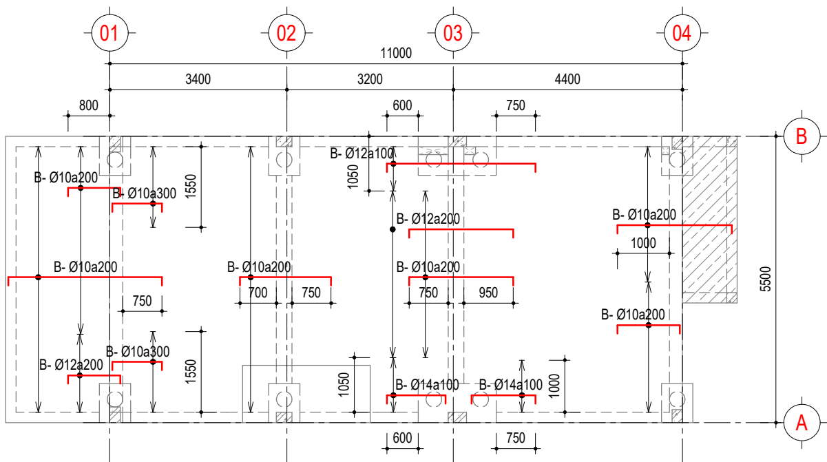
MẶT BẰNG THÉP SÀN TẦNG 1-LỚP TRÊN PHƯƠNG X
