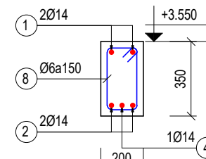
MC 10-10 2X1 (TL: 1/25)
