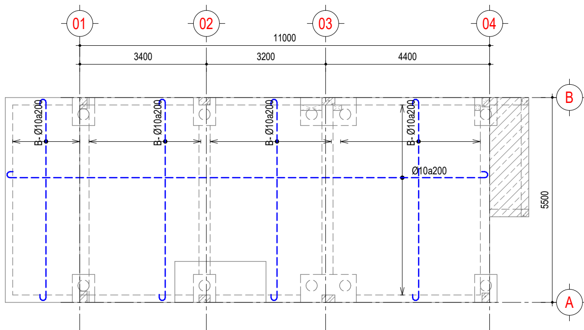
MẶT BẰNG THÉP SÀN TẦNG 1-LỚP DƯỚI
