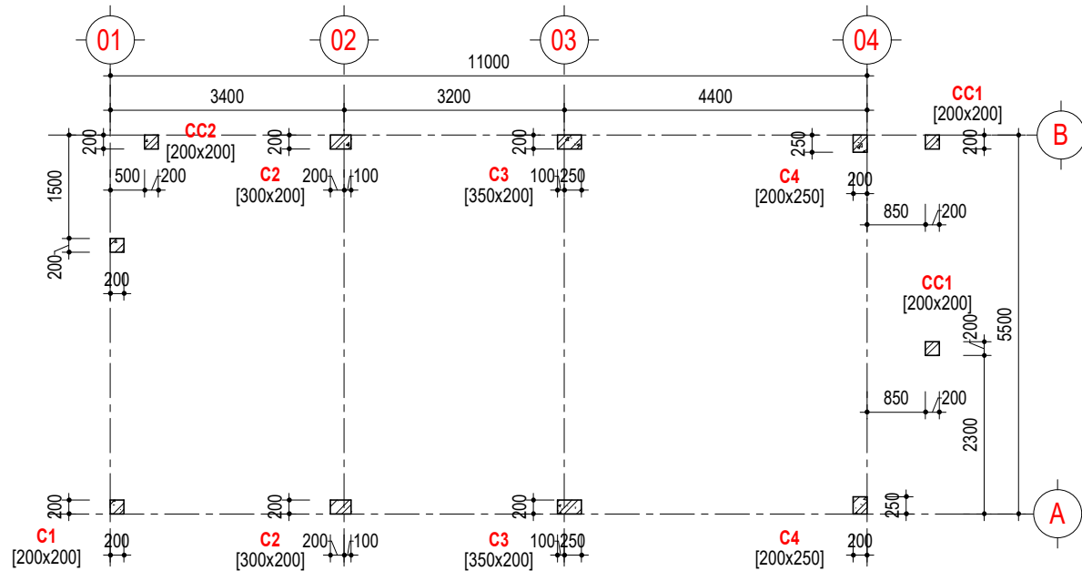
MẶT BẰNG CỘT - TẦNG 2
