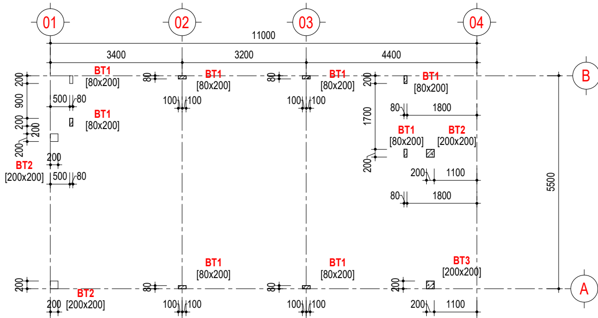
MẶT BẰNG CỘT - MÁI
