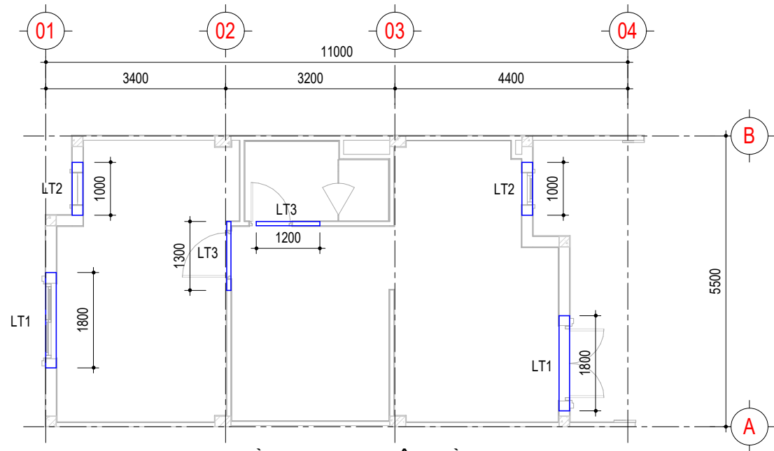
MẶT BẰNG LANH TÔ - TẦNG 3 TL 1 : 100
