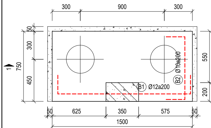
MÓNG M3 (SL=1)
