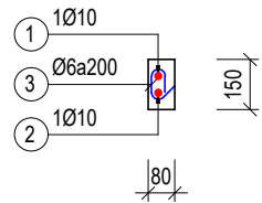
DẪN LT3 (SL=1; L=8600) TL: 1/25
