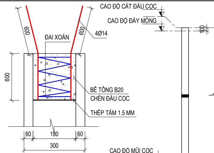
CHI TIẾT ĐỈNH CỌC TỈ LỆ: 1/10
