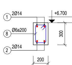
MC 4-4 3X1 (TL: 1/25)
