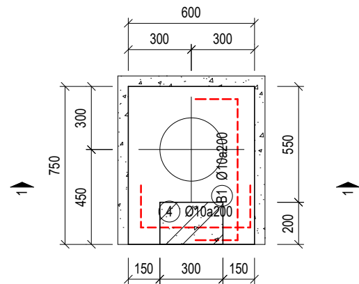
MÓNG M2 (SL=2)
