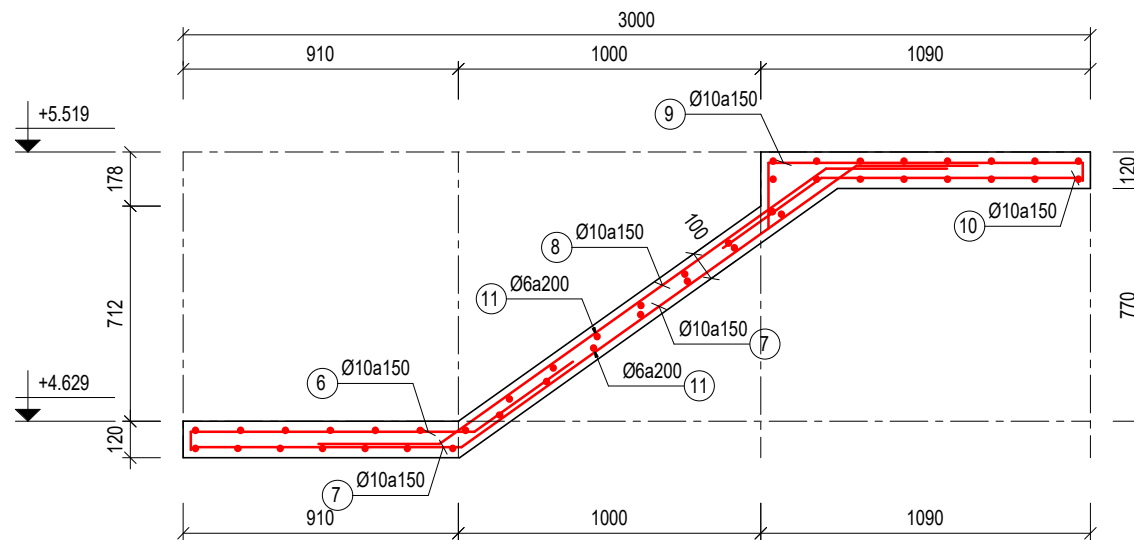
THANG BỘ TẦNG 2 (MC B-B)
