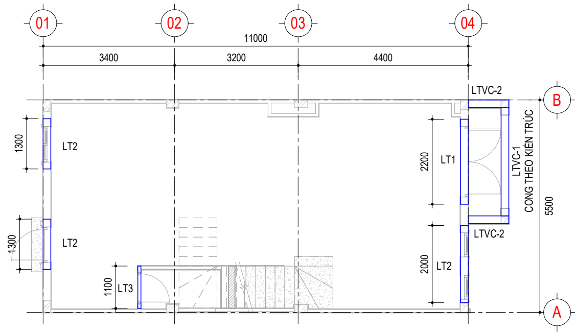
MẶT BẰNG LANH TÔ - TẦNG 1 TL 1 : 100
