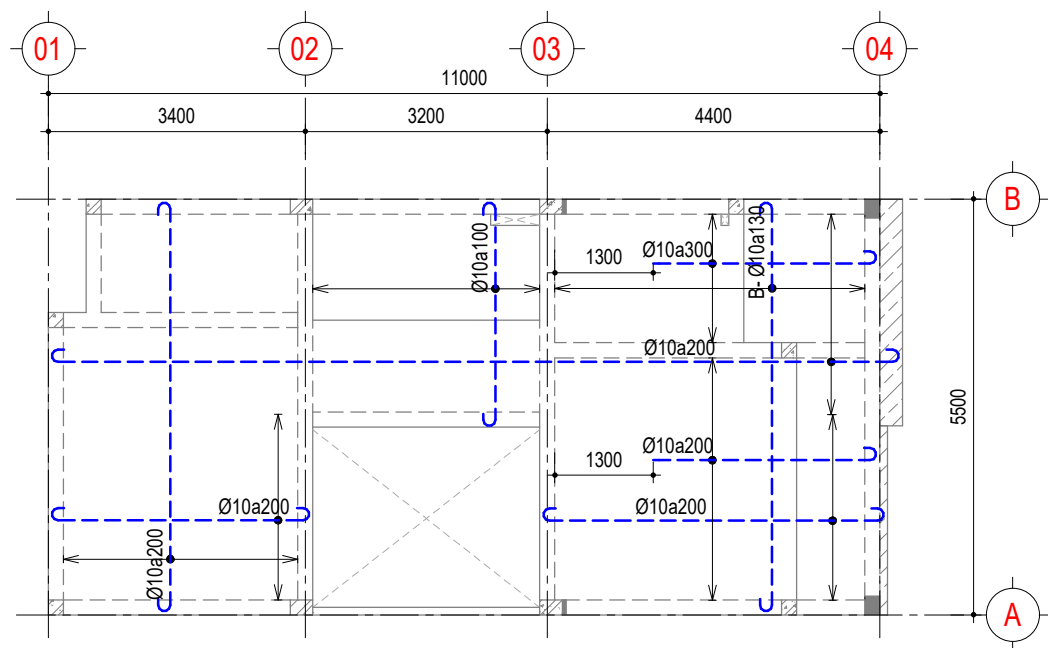
MẶT BẰNG THÉP SÀN TẦNG 3-LỚP DƯỚI
