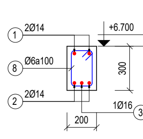
MC 10-10 3X1 (TL: 1/25)
