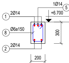
MC 3-3 3X1 (TL: 1/25)
