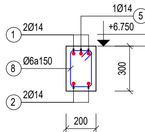
MC 2-2 3X1 (TL: 1/25)
