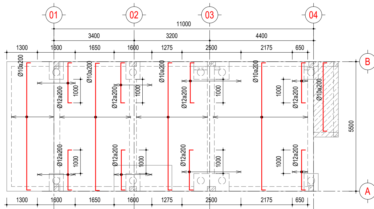
MẶT BẰNG THÉP SÀN TẦNG 1-LỚP TRÊN PHƯƠNG Y
