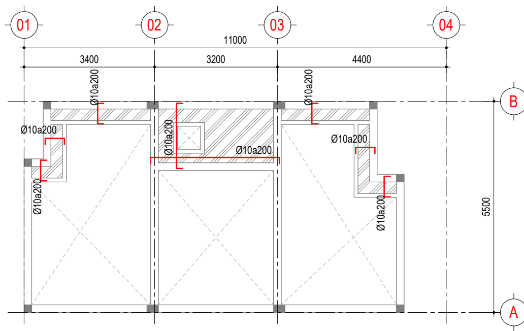
MẶT BẰNG THÉP SÀN MÁI-LỚP TRÊN
