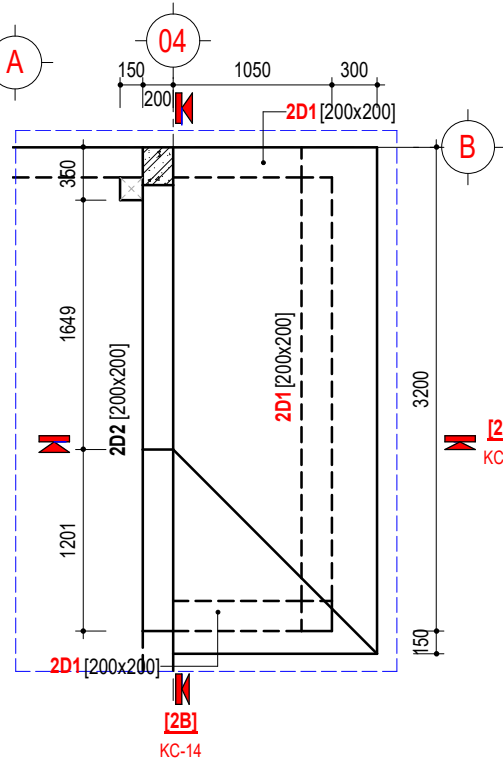
MẶT BẰNG MÁI XIÊN - TẦNG 2
