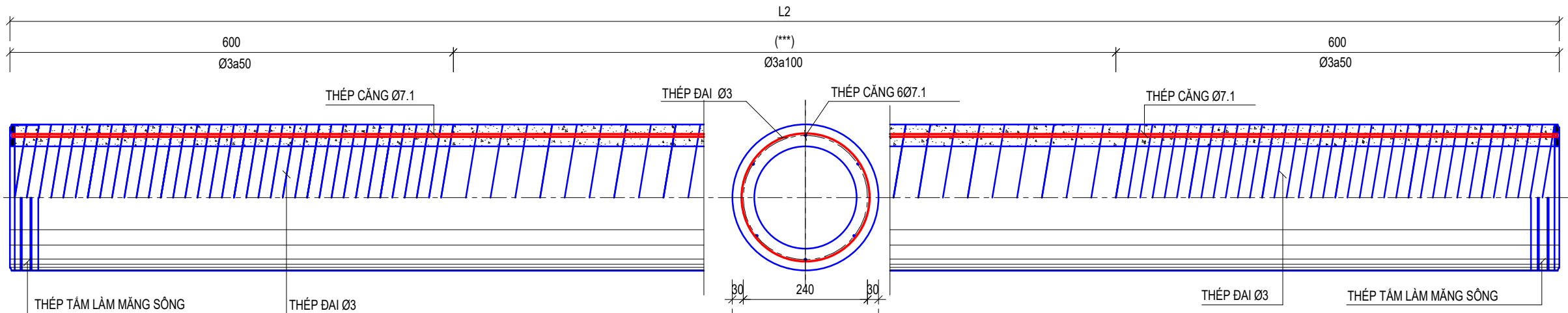
ĐOẠN CỌC 2
