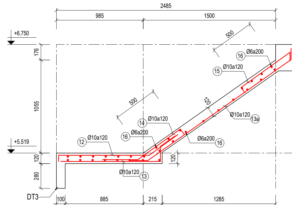
THANG BỘ TẦNG 2 (MC C-C)
