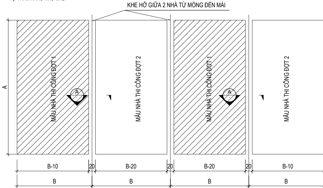
MẶT BẰNG TRÍCH ĐOẠN PHÂN ĐOẠN THI CÔNG ĐIỂN HÌNH
