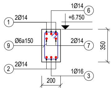
MC 6-6 3X1 (TL: 1/25)
