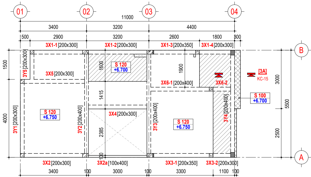
MẶT BẰNG DẦM SÀN - TẦNG 3
