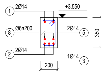
MC 2-2 2X1 (TL: 1/25)
