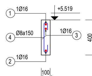
DÀM DT3 (SL=1; L=1390)
