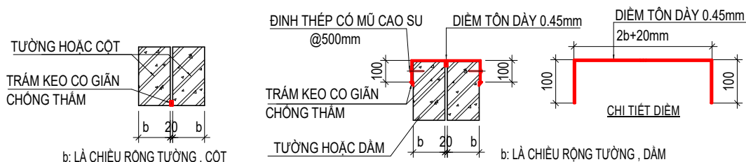
VI TRÍ MẶT ĐỨNG, MẶT NGHIẾNG GIỮA 2 NHÀ
