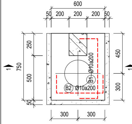
MÓNG M4 (SL=2)
