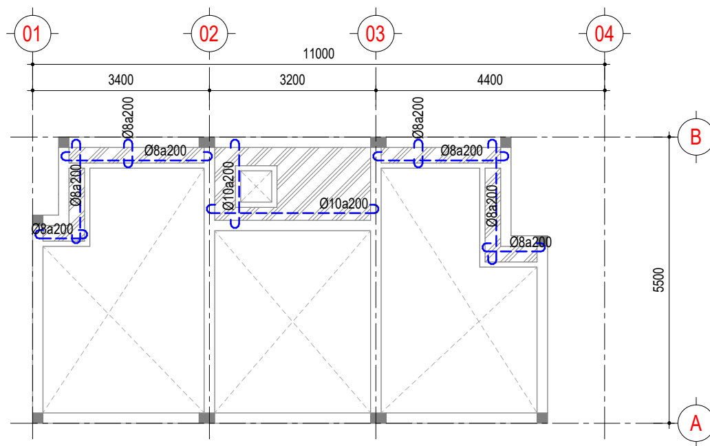
MẶT BẰNG THÉP SÀN MÁI-LỚP DƯỚI
