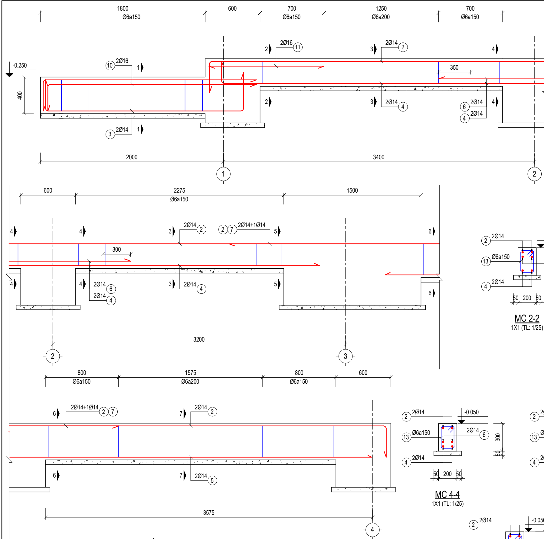
DẦM 1X1 (SL=1; L=13200) TL: 1/25
