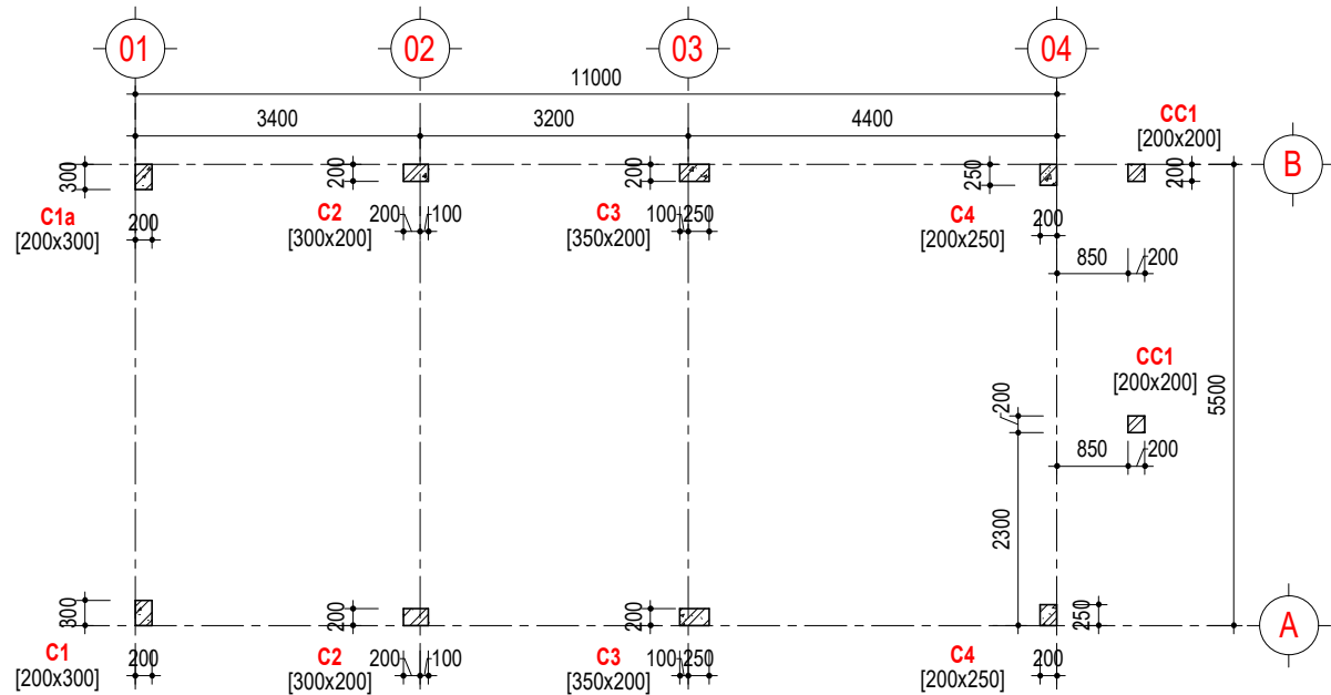
MẶT BẰNG CỘT - TẦNG 1
