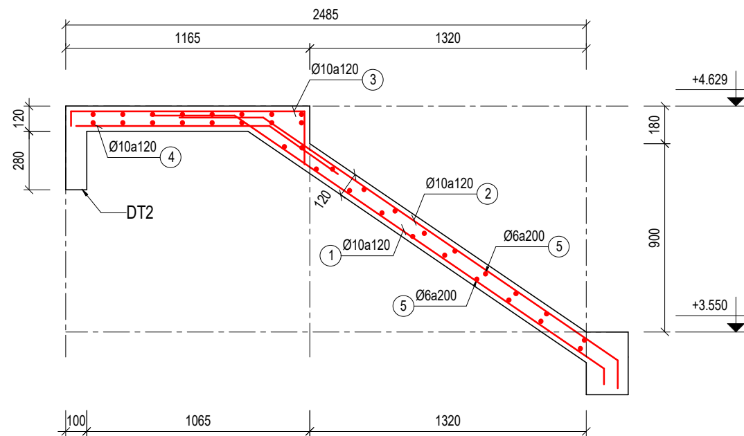
THANG BỘ TẦNG 2 (MC A-A)
