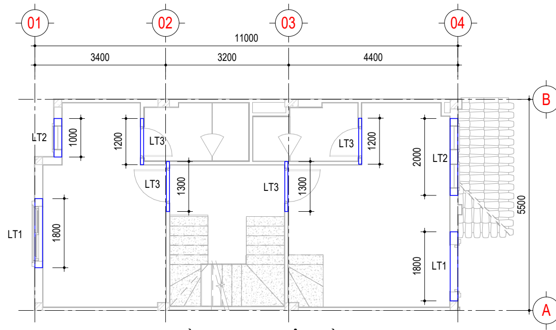
MẶT BẰNG LANH TÔ - TẦNG 2 TL 1 : 100
