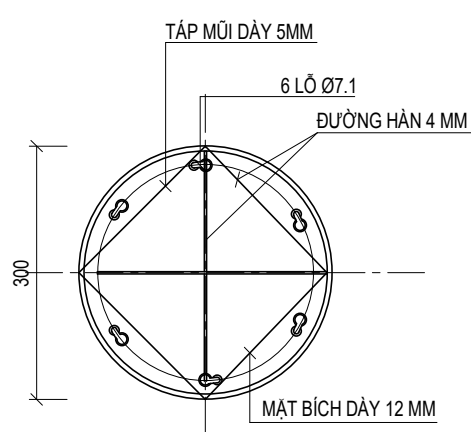
CHI TIẾT ĐỈNH CỌC TỈ LỆ: 1/10
