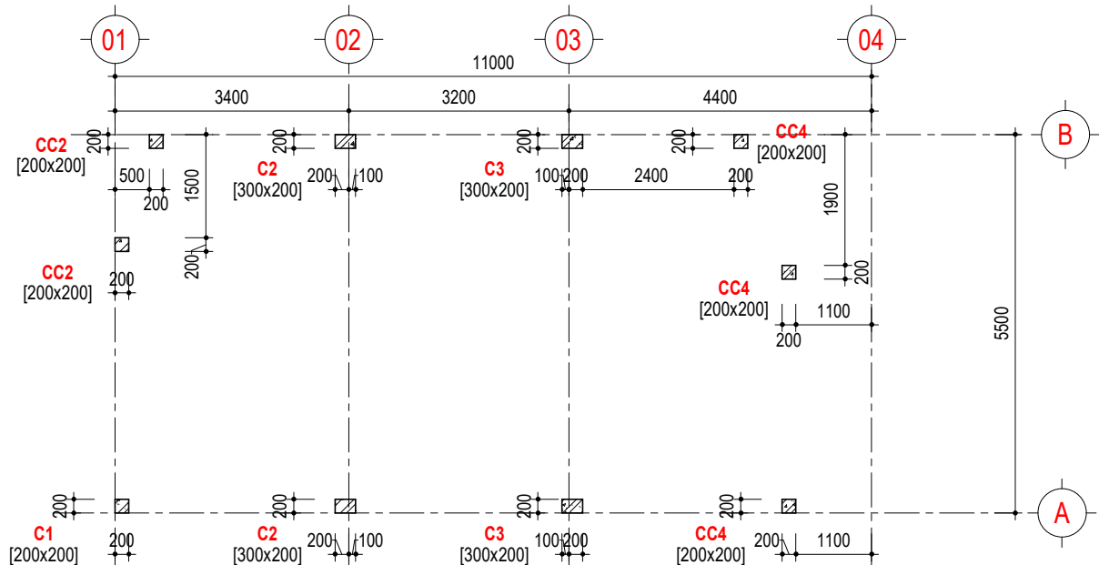
MẶT BẰNG CỘT - TẦNG 3
