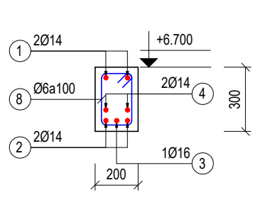
MC 9-9 3X1 (TL: 1/25)
