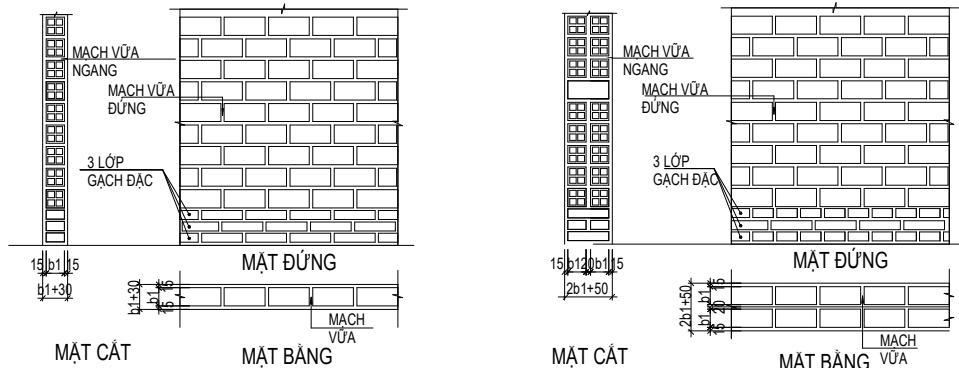
TƯỜNG ĐƠN DÀY <150
