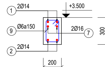
MC 7-7 2X1 (TL: 1/25)
