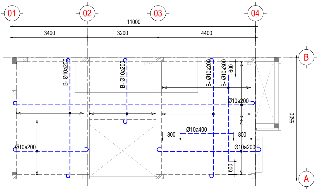
MẶT BẰNG THÉP SÀN TẦNG 2-LỚP DƯỚI
