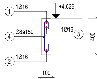
DÀM DT2 (SL=1; L=1350)
