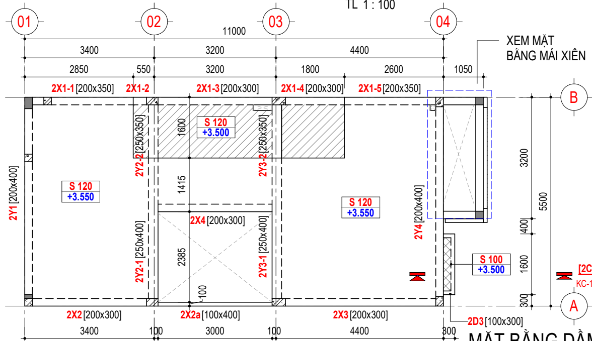
MẶT BẰNG DẦM SÀN - TẦNG 2
